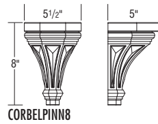
8" PINNACLE CORBEL R•26
