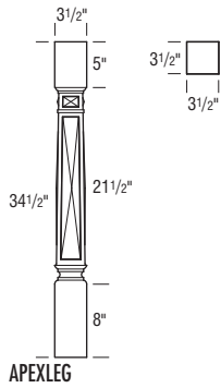
APEX LEG R•41
