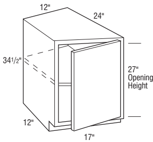
Left Angle Shown
